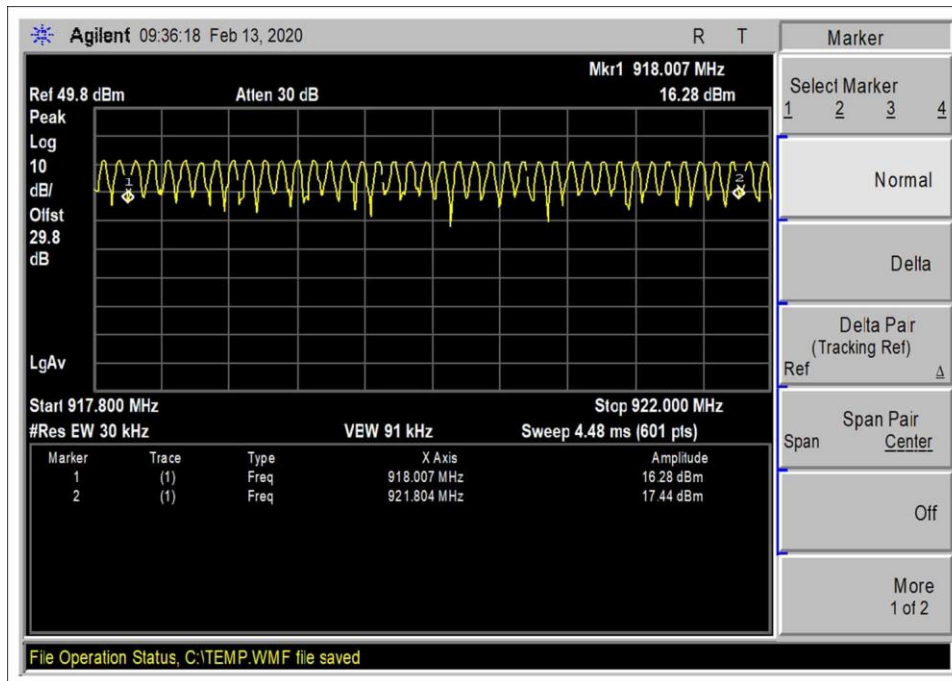
918-921.8MHz - 20 Channel
