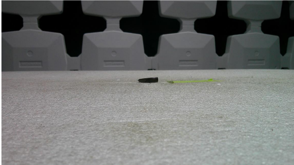
Band Edge
