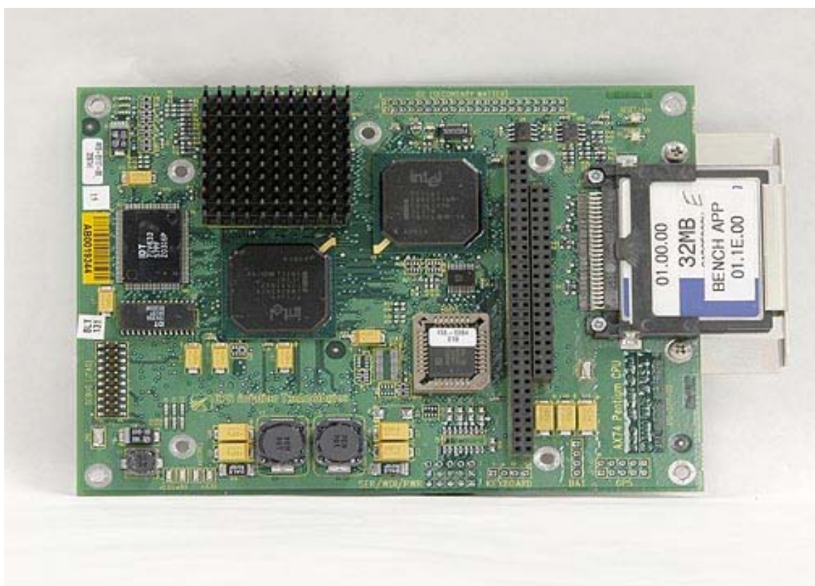
DSP 2
