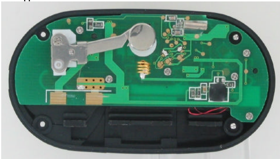
Antenna
