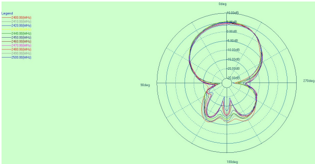
2.4G phi=0deg
