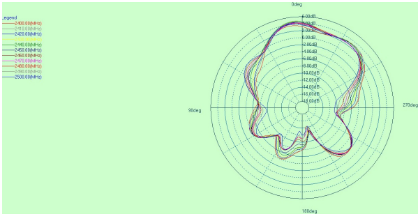
2.4G phi=0deg
