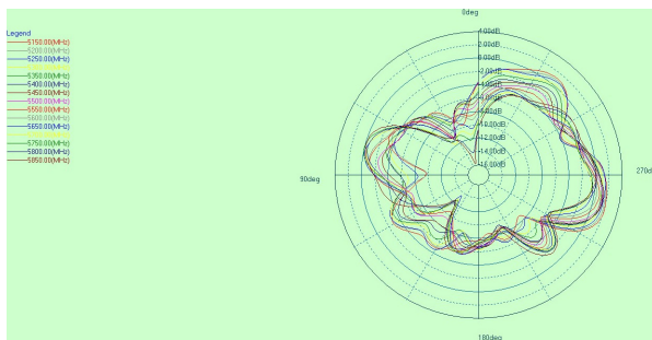
5G theta=90deg
