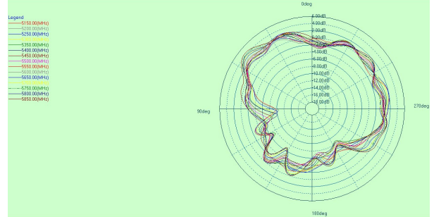
5G phi=90deg
