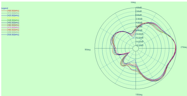
2.4G theta=90deg
