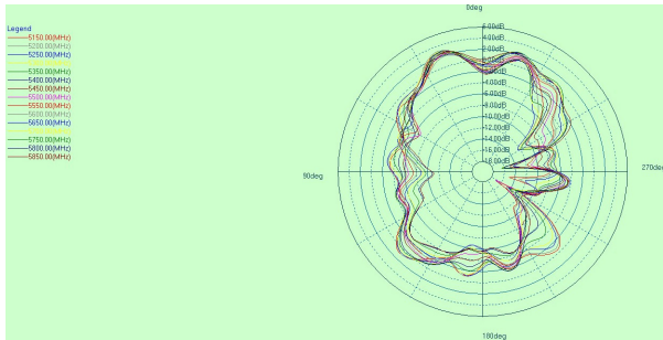
5G phi=0deg
