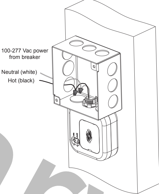
ZUMMESH-JBOX-PSU Wiring
