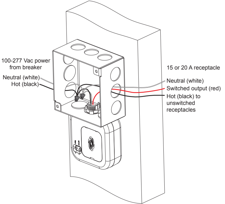
ZUMMESH-JBOX-PSU Wiring
