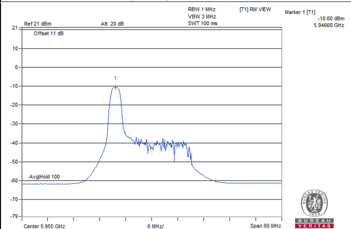
802.11ax (HE20) 26-tone RU / Chain 0 : CH 1@0
