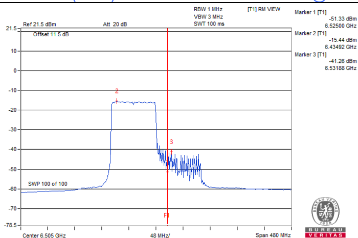
802.11ax (HE160) 996-tone RU / Chain 1 : CH 111@67
