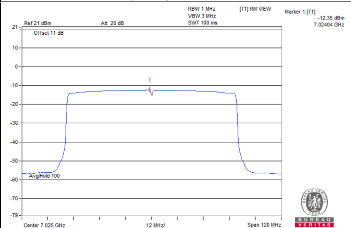
802.11ax (HE80) / Chain 1 : CH 215
