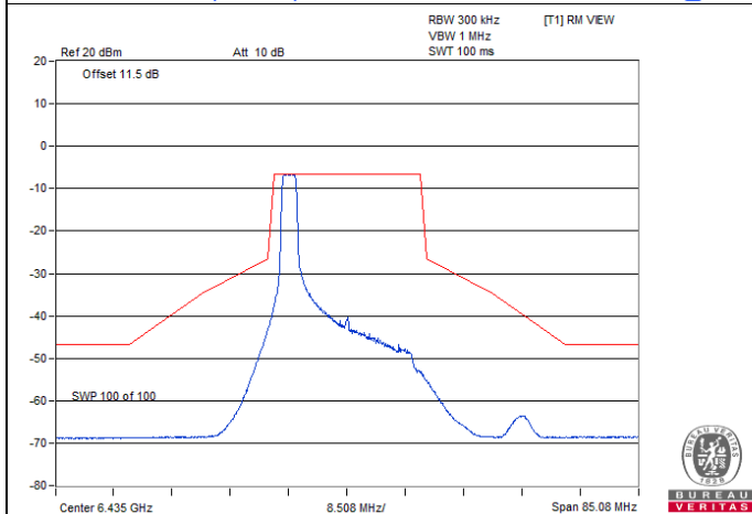
802.11ax (HE20) 26-tone RU / Chain 1 : CH 97@0
