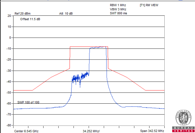
802.11ax (HE80) 484-tone RU / Chain 0 : CH 119@66
