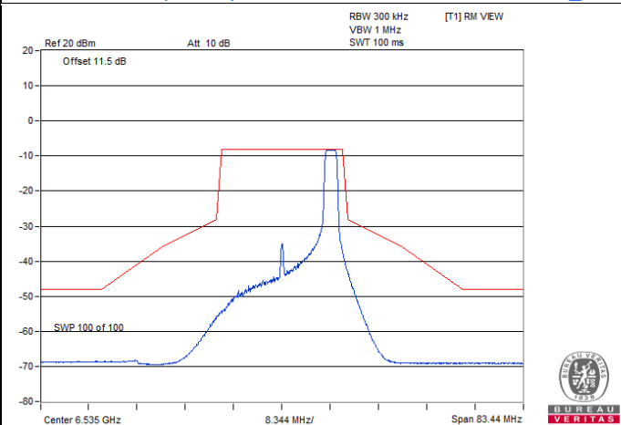
802.11ax (HE20) 26-tone RU / Chain 1 : CH 117@0
