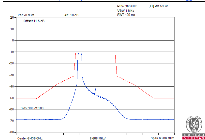
802.11ax (HE20) 26-tone RU / Chain 0 : CH 97@0
