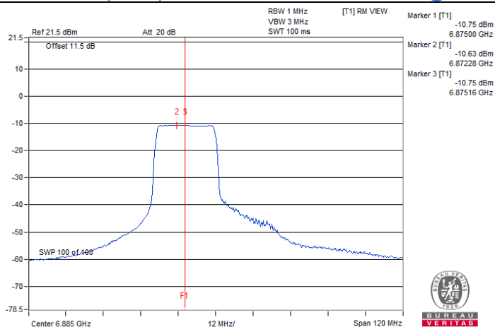
802.11ax (HE40) 242-tone RU / Chain 0 : CH 187@61
