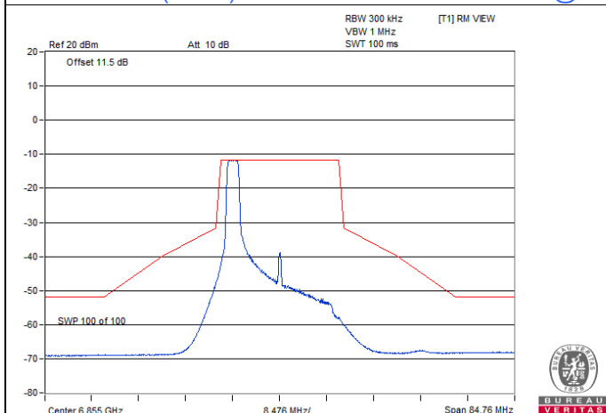
802.11ax (HE20) 26-tone RU / Chain 1 : CH 181@8
