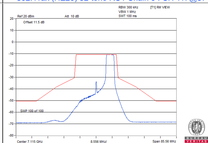
802.11ax (HE20) 52-tone RU / Chain 0 : CH 233@40
