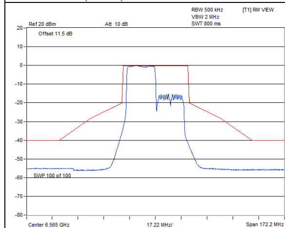
802.11ax (HE40) 242-tone RU / Chain 0 : CH 123@61
