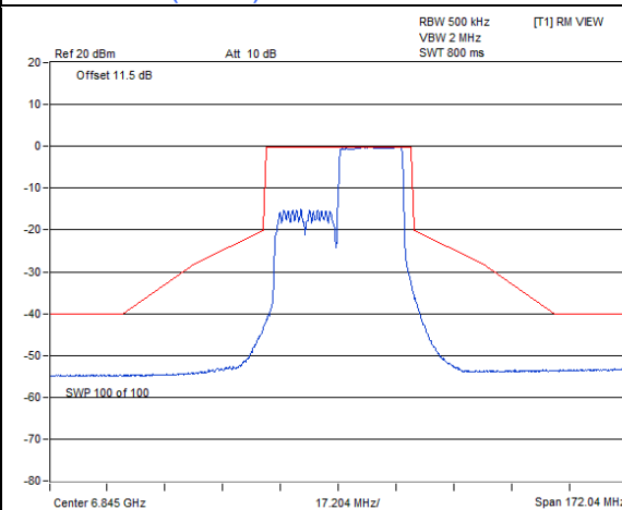
802.11ax (HE40) 242-tone RU / Chain 0 : CH 179@62
