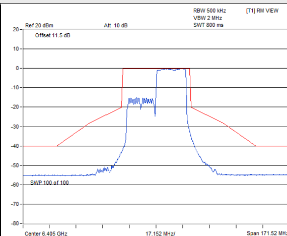
802.11ax (HE40) 242-tone RU / Chain 0 : CH 91@62
