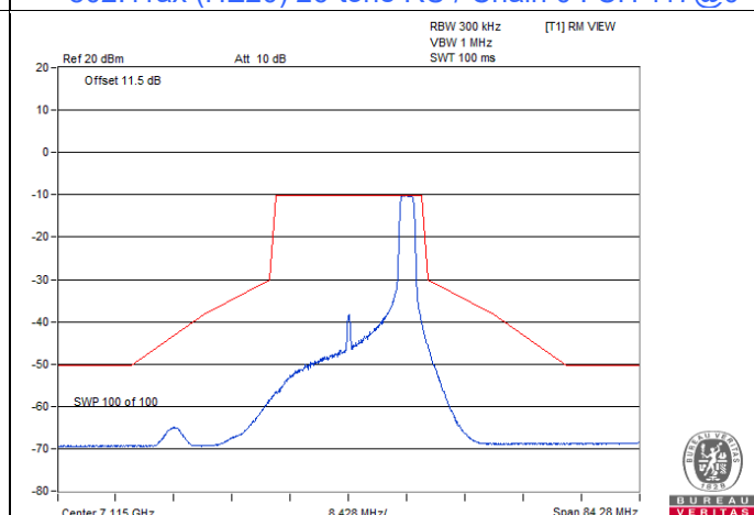
802.11ax (HE20) 26-tone RU / Chain 0 : CH 233@8
