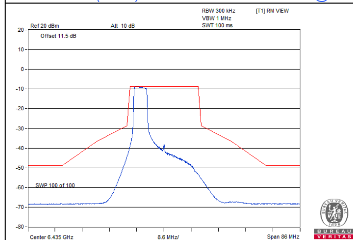
802.11ax (HE20) 52-tone RU / Chain 0 : CH 97@37
