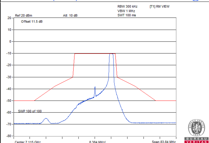
802.11ax (HE20) 26-tone RU / Chain 1 : CH 233@8
