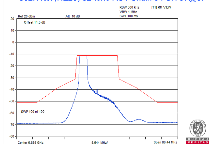
802.11ax (HE20) 52-tone RU / Chain 0 : CH 181@40
