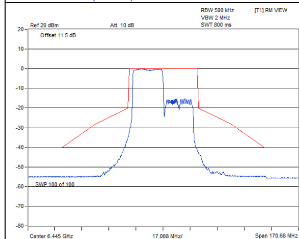
802.11ax (HE40) 242-tone RU / Chain 0 : CH 99@61
