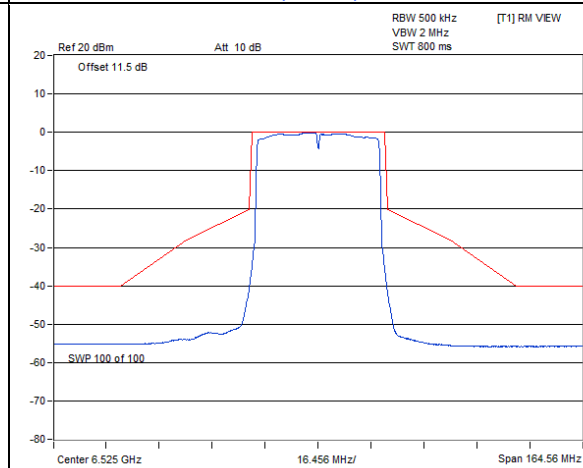
802.11ax (HE40) / Chain 0 : CH 115
