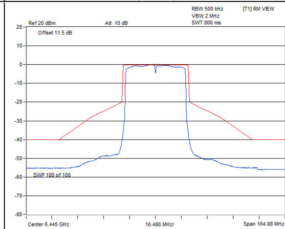
802.11ax (HE40) / Chain 0 : CH 99
