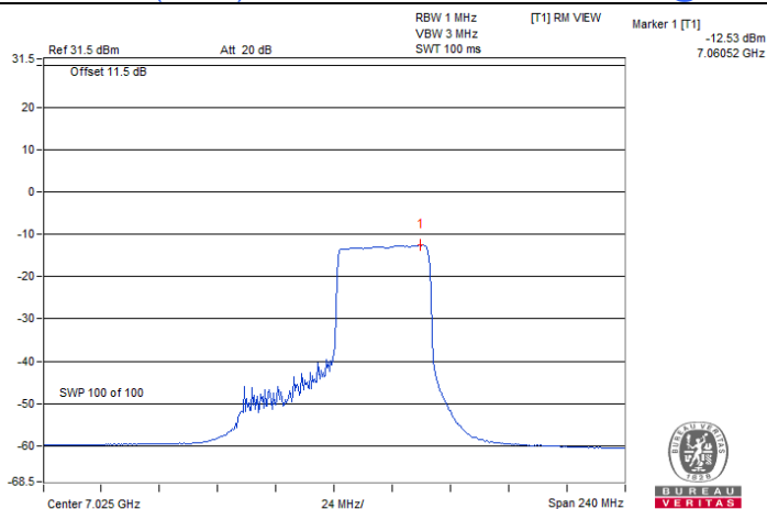
802.11ax (HE80) 484-tone RU / Chain 1 : CH 215@66
