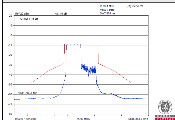
802.11ax (HE80) 484-tone RU / Chain 0 : CH 7@65
