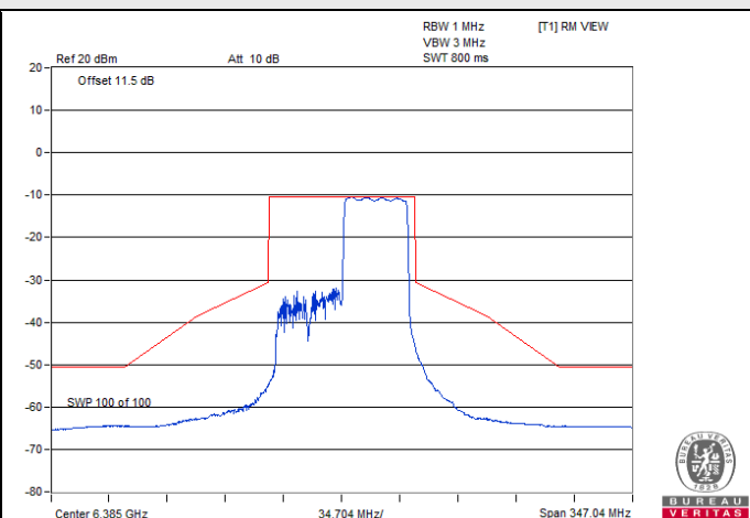
802.11ax (HE80) 484-tone RU / Chain 0 : CH 87@66
