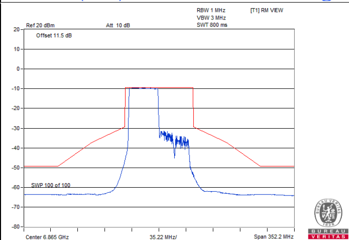
802.11ax (HE80) 484-tone RU / Chain 0 : CH 183@65
