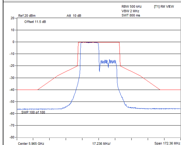
802.11ax (HE40) 242-tone RU / Chain 0 : CH 3@61
