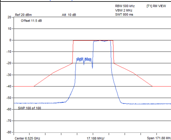
802.11ax (HE40) 242-tone RU / Chain 0 : CH 115@62
