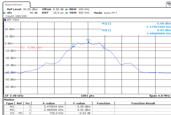
LE 1M_Ant1_2480
