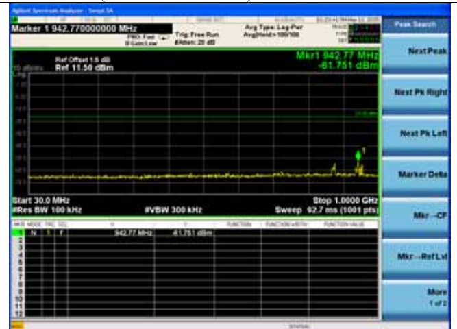
2402MHz(30MHz – 1GHz)
