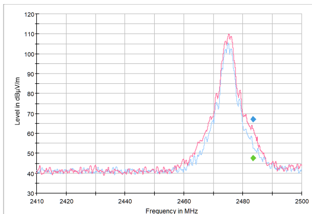
Figure 3. Band Edge
