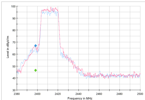
Figure 10. Band Edge
