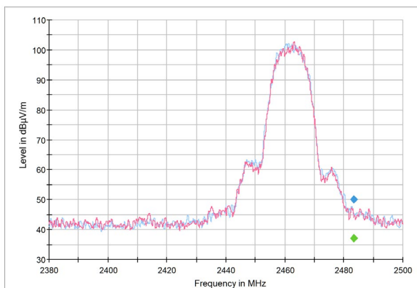
Figure 3. Band Edge
