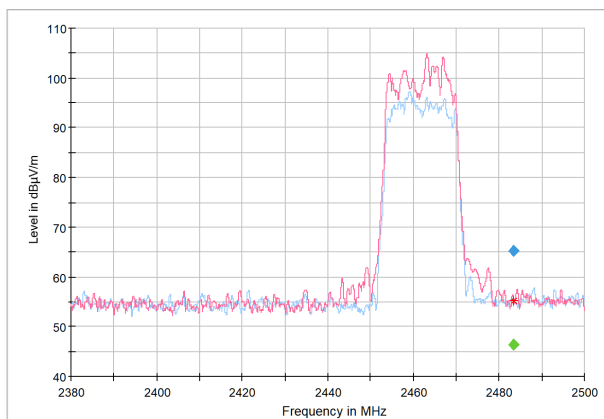
Figure 9. Band Edge
