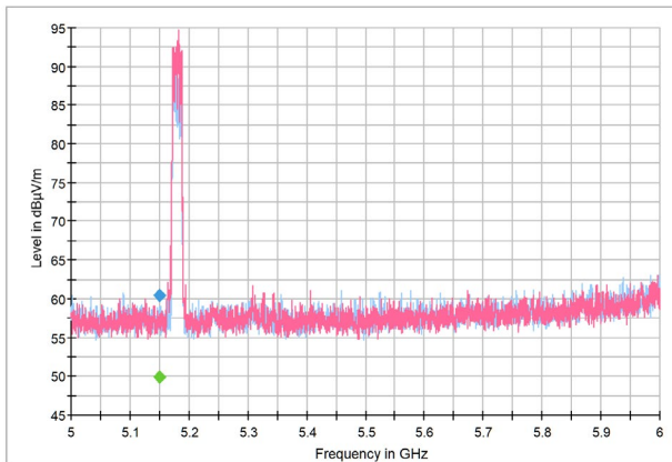
Figure 3. Band Edge
