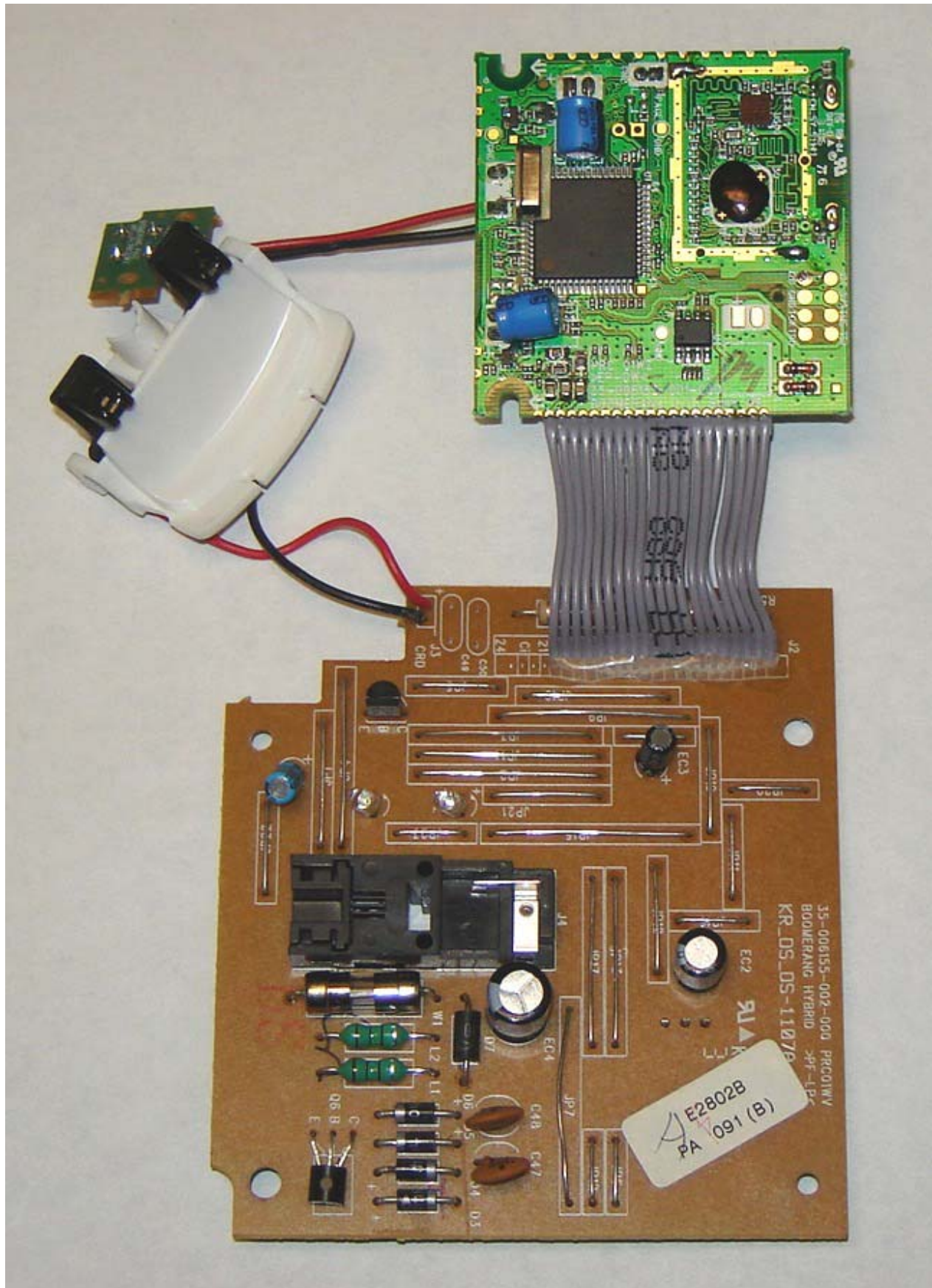
AT&T E2801 BS PCB
