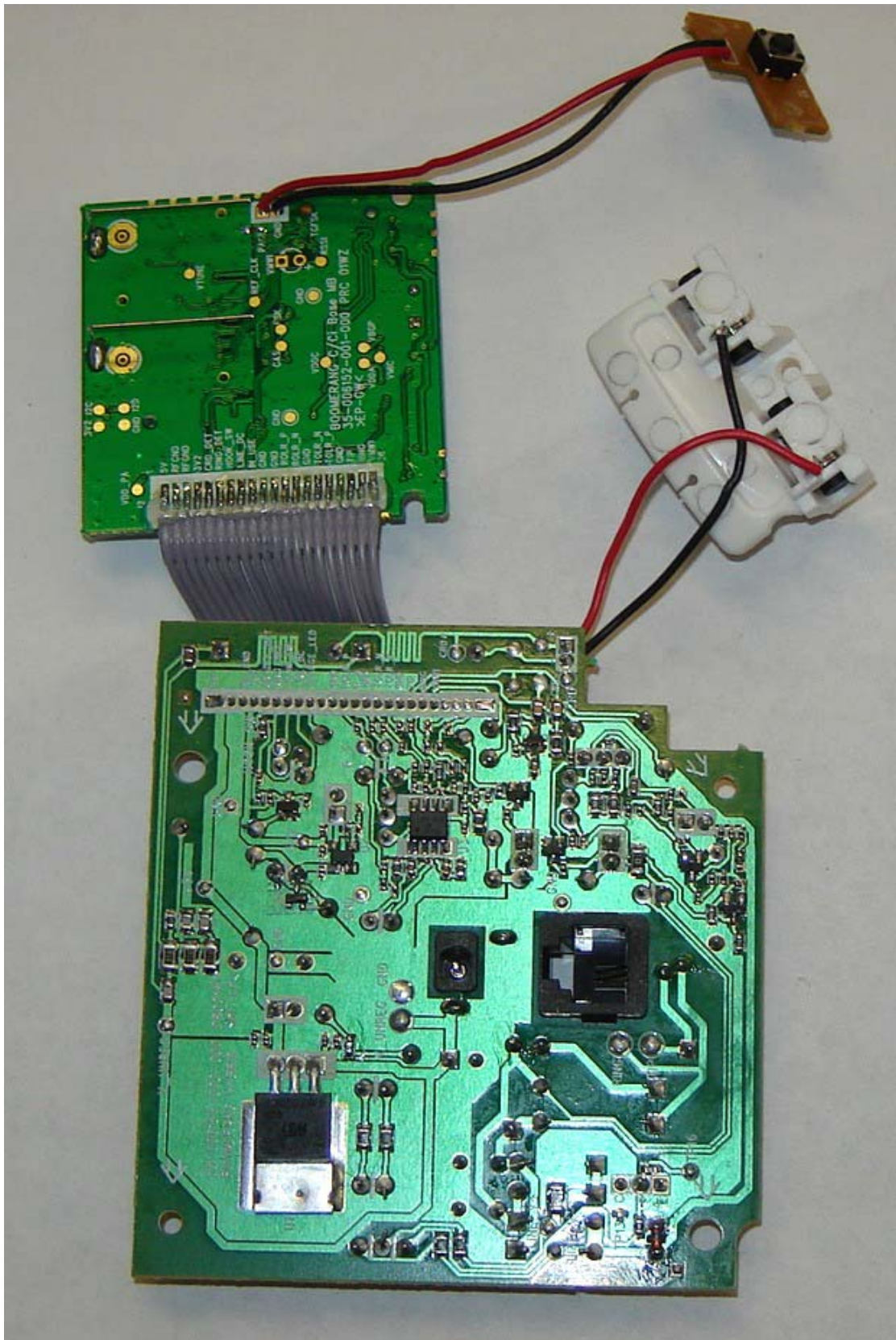
AT&T E2801 Base PCB
