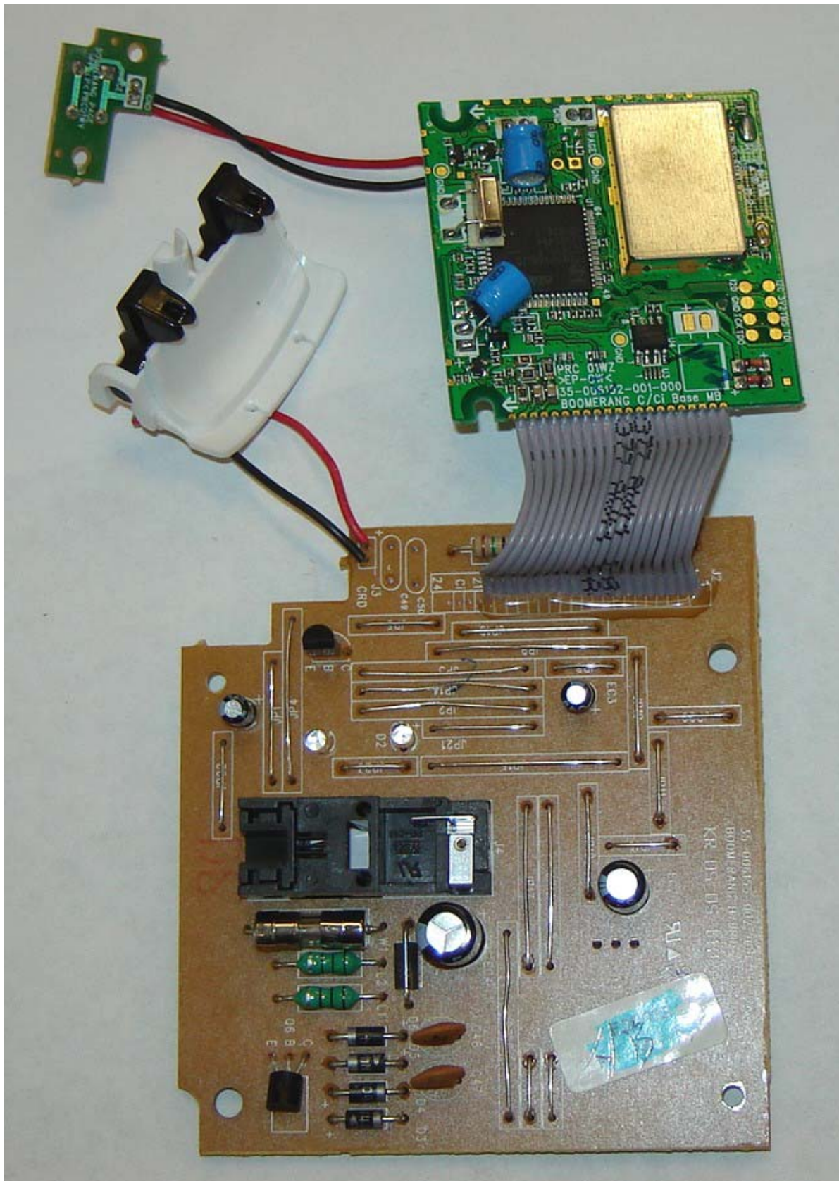
AT&T E2801 Base PCB
