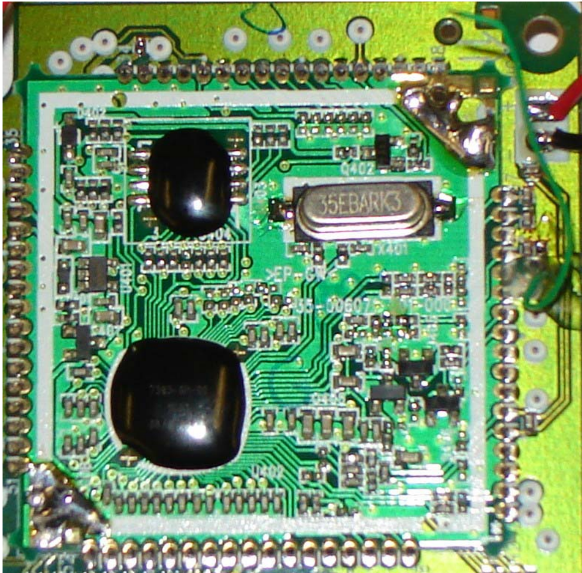
AT&T E2811 Base RF PCB
