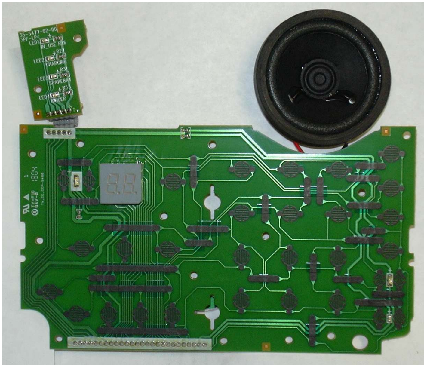
AT&T E2135 Base PCB
