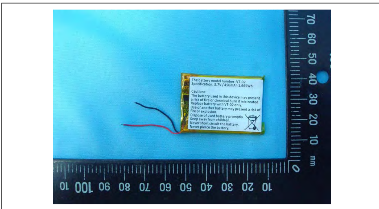
EUT Photo ( 3 )
