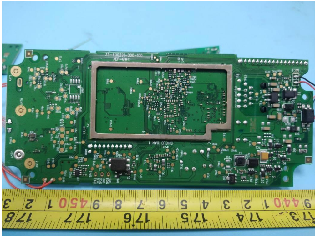
IC Chip
