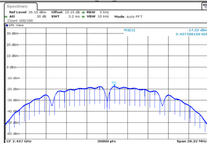
11B_Ant1_2437
