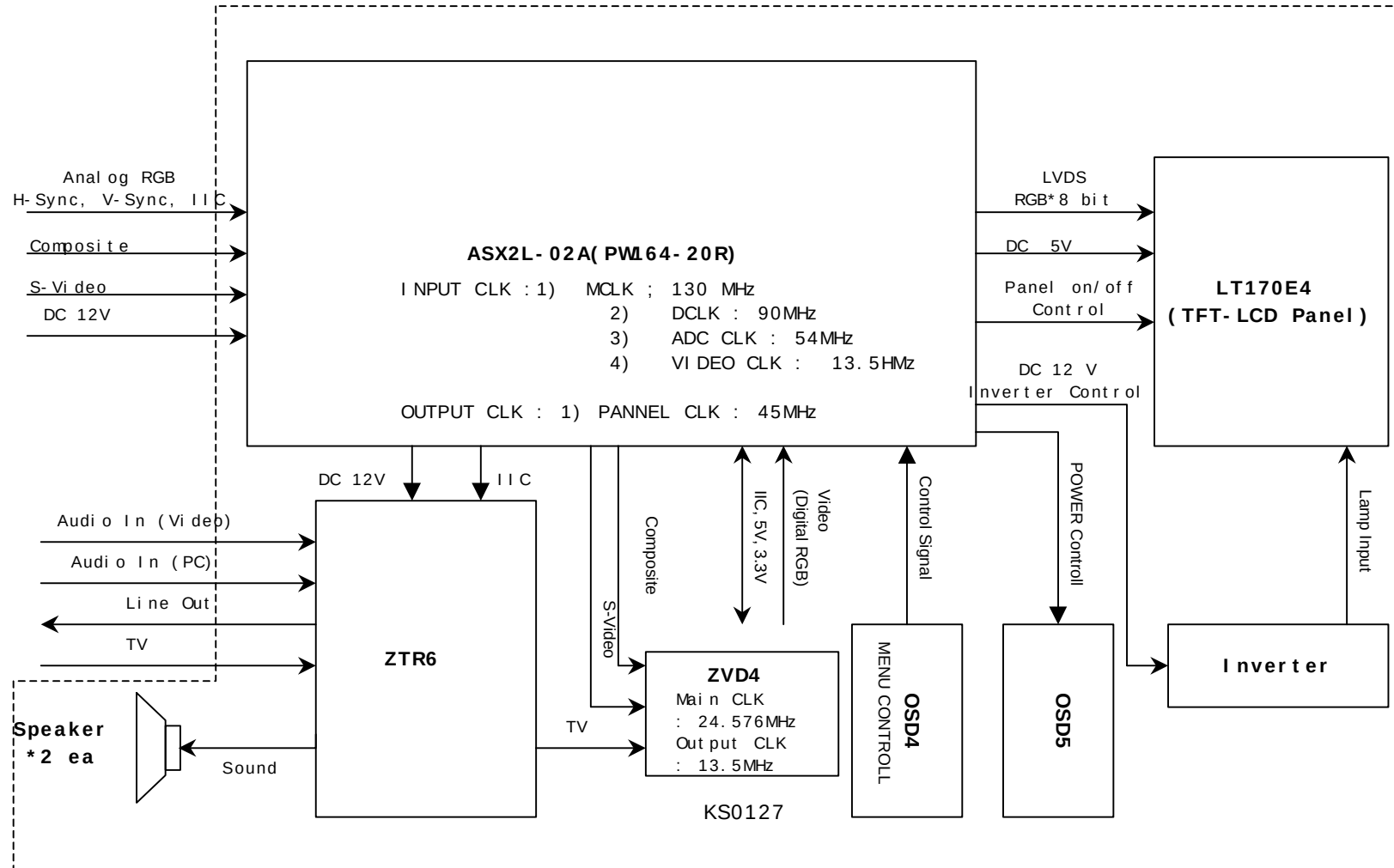
LN710S TFT- LCD Moni t or Bl ock Di agram
