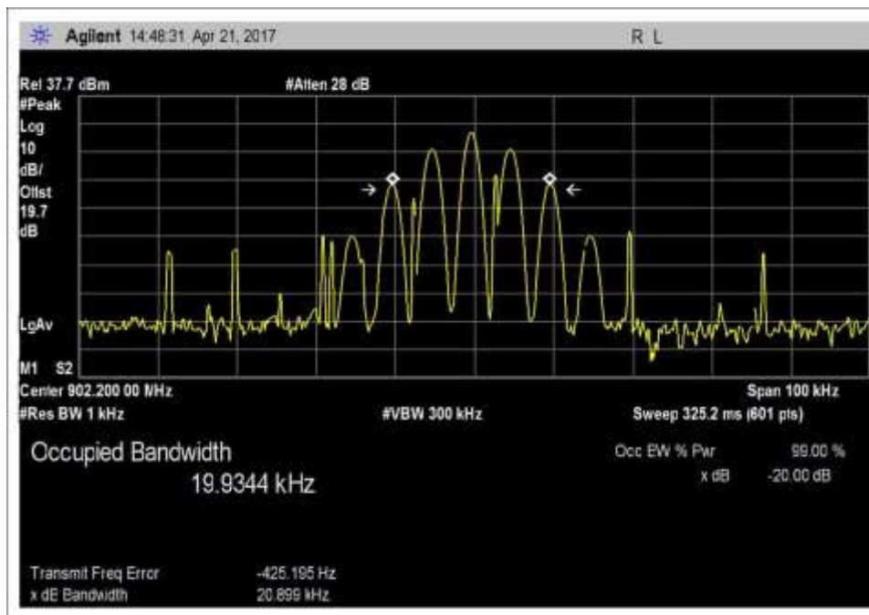
20dB_99%BW_902.2MHz_27dBm_10kbps
