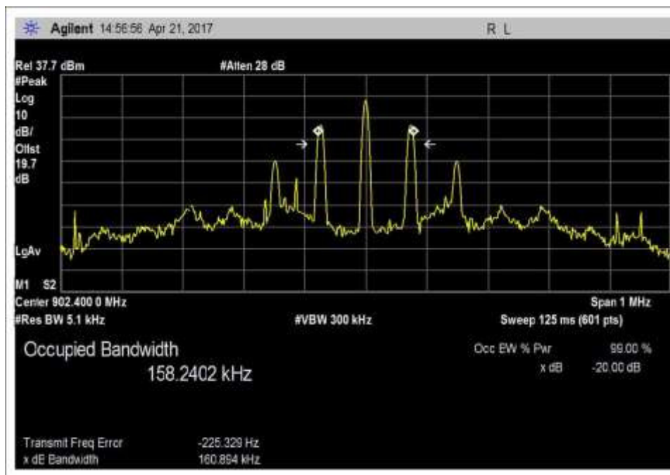
20dB_99%BW_902.4MHz_27dBm_150kbps
