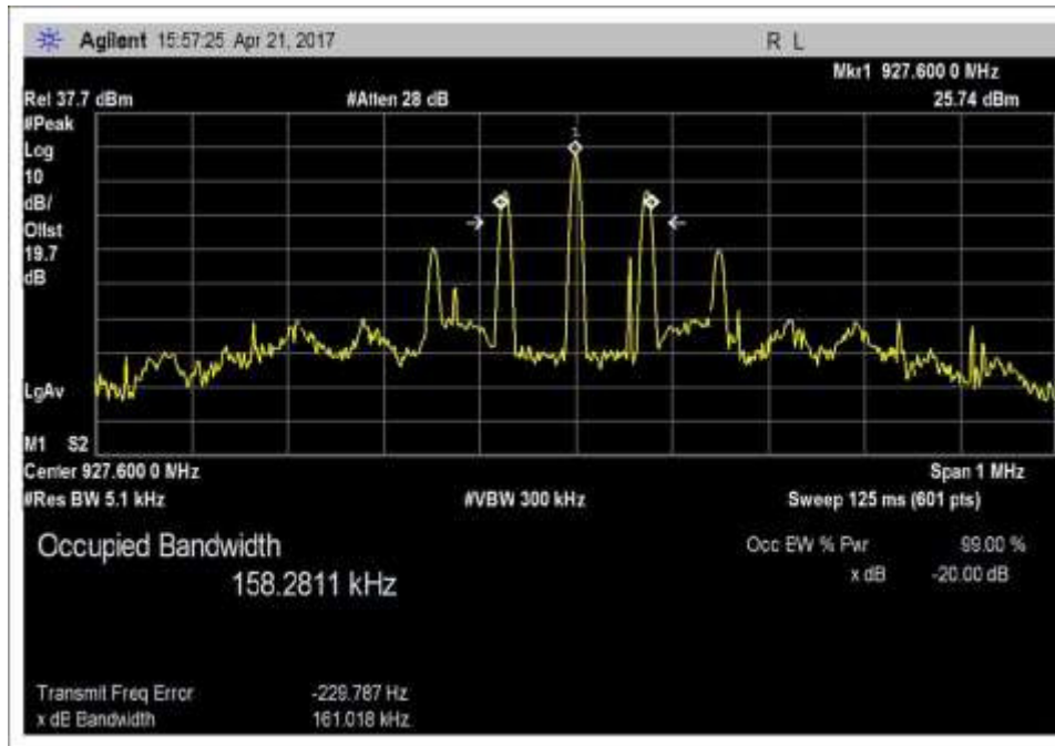
20dB_99%BW_927.6MHz_27dBm_150kbps
