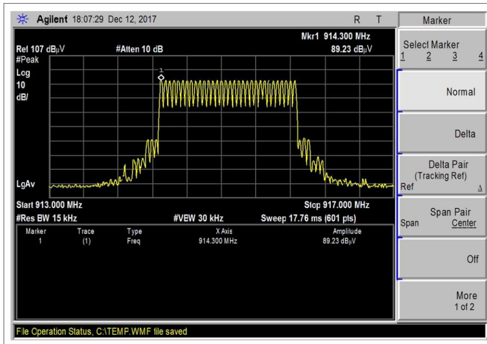
GFSK_10kbps_Middle_32CH
