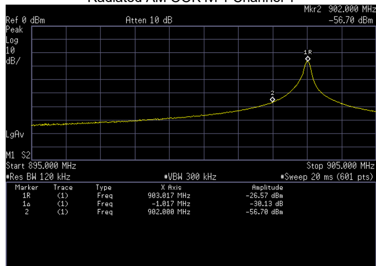
Radiated AM OOK lvl 1 Channel 1
