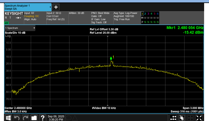
2Mbps / 2480MHz
