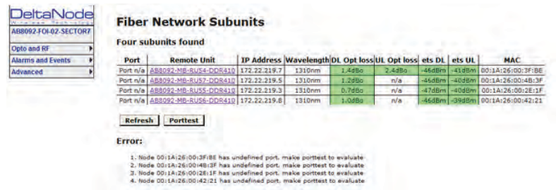
Figure 89 DOI401 FOI Fiber Network Subunits
