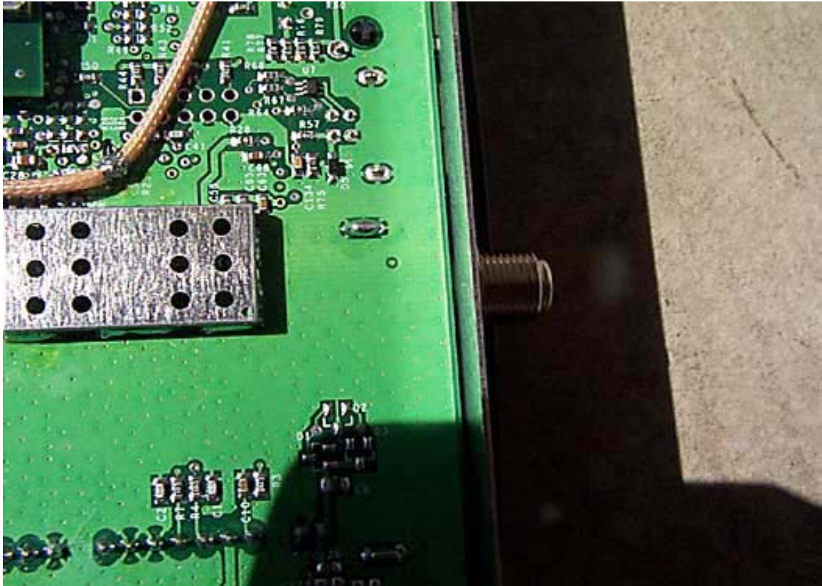
SBG900 Antenna 1
