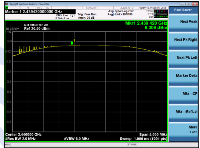
PWR -Zigbee 2440
