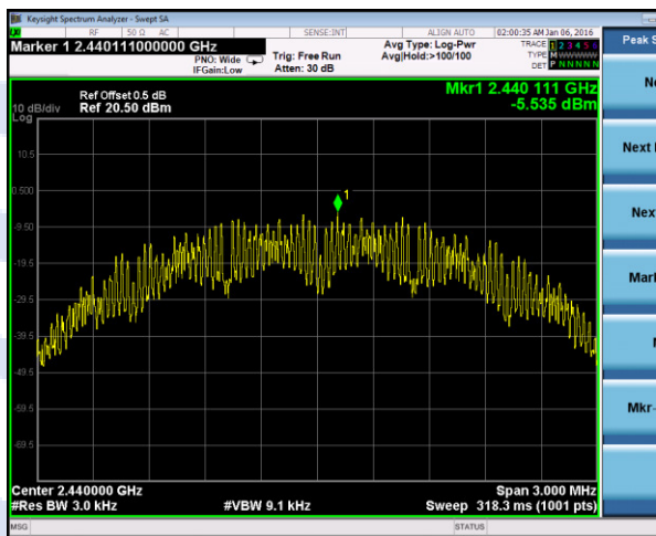
2440MHz PSD
