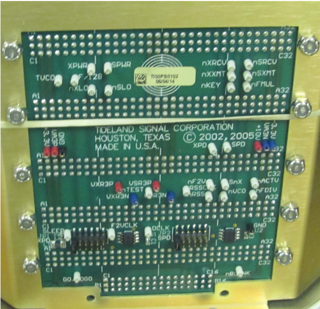
Backplane
