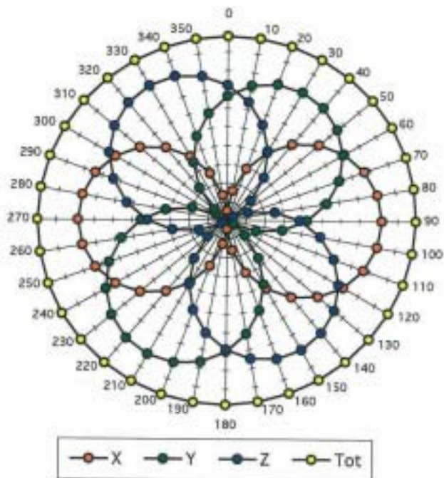
f = 30 \text{ MHz} , TEM cell if110
