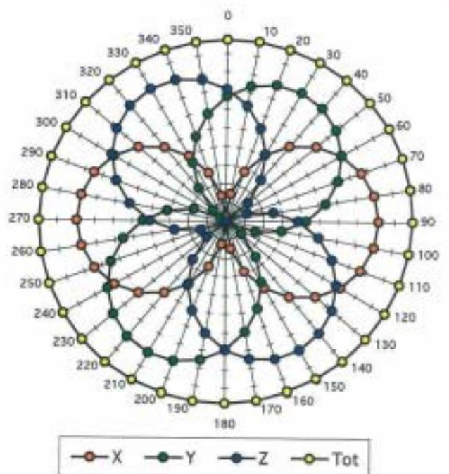
f = 900 \text{ MHz} , TEM cell if110
