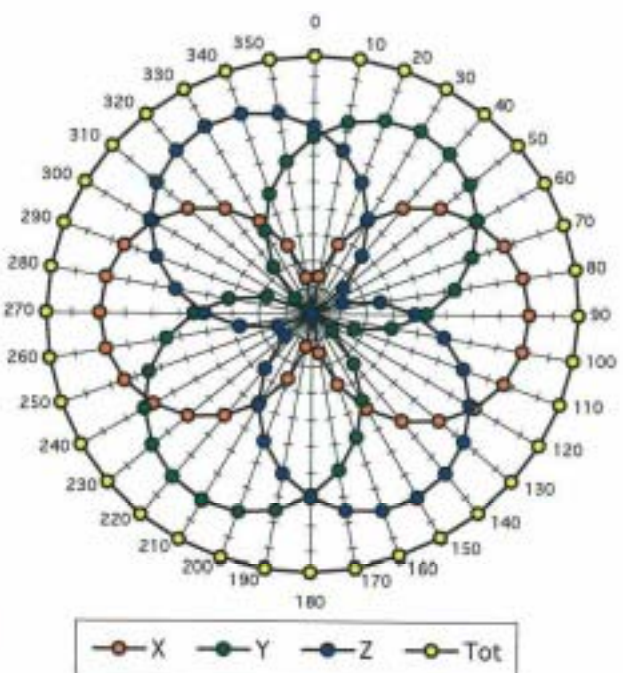
f = 300 \text{ MHz} , TEM cell if110
