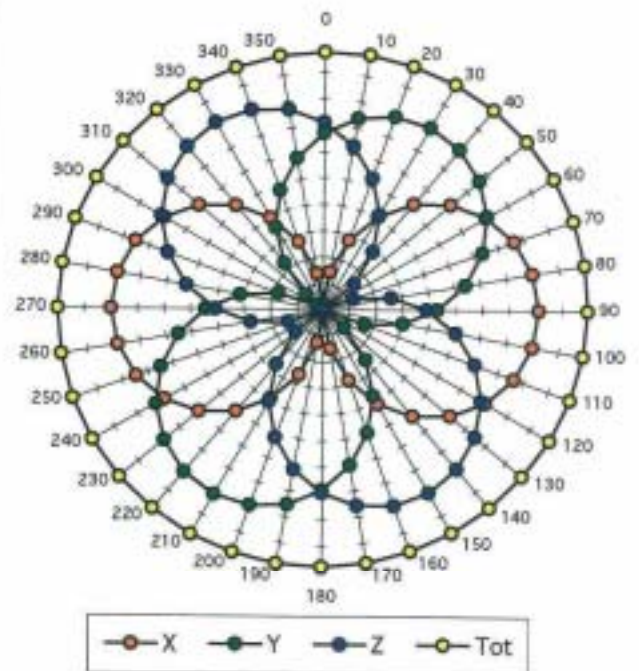
f = 100 \text{ MHz} , TEM cell if110
