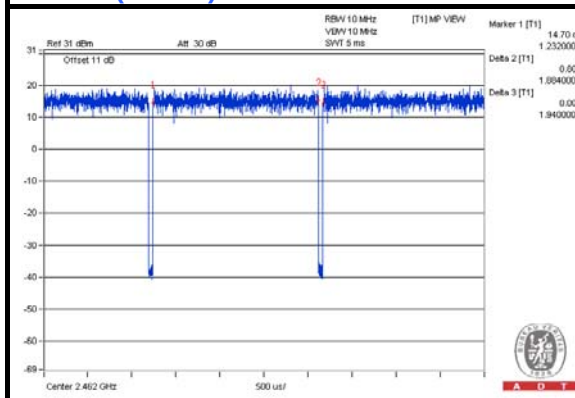
802.11n (20MHz)
