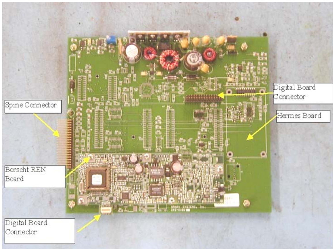
HERMES and BORSCHT REN BOARD
