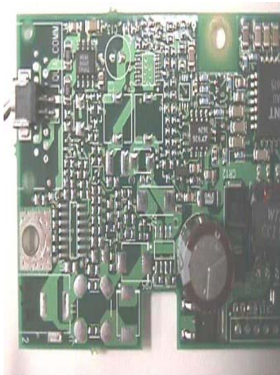
BORSCHT REN CARD ZOOM
