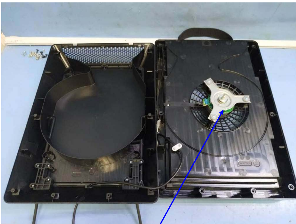
Fan motor location
