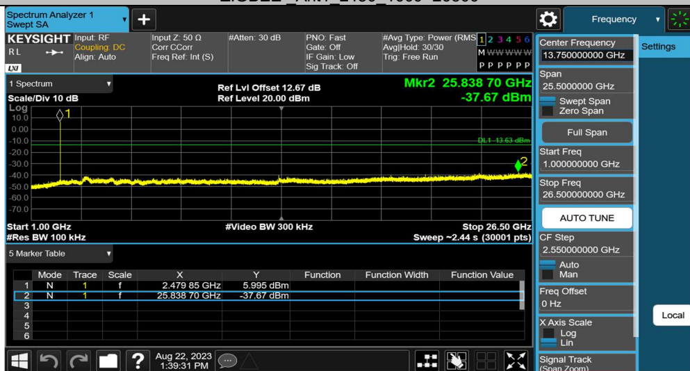
ZIGBEE Ant1 2480 1000~26500
