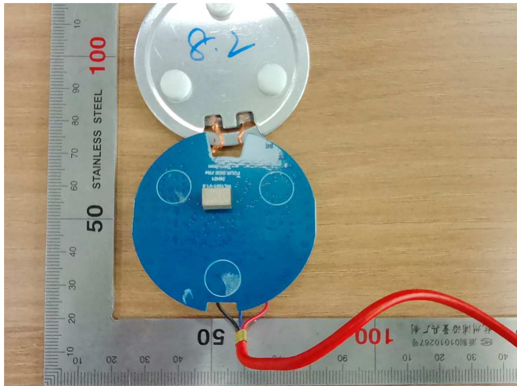
Bild / Picture 4: PCB view
