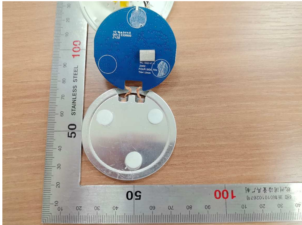
Bild / Picture 3: PCB view
