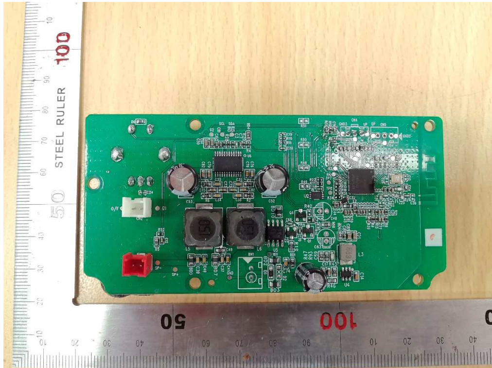
Bild / Picture 4: Mainboard view
