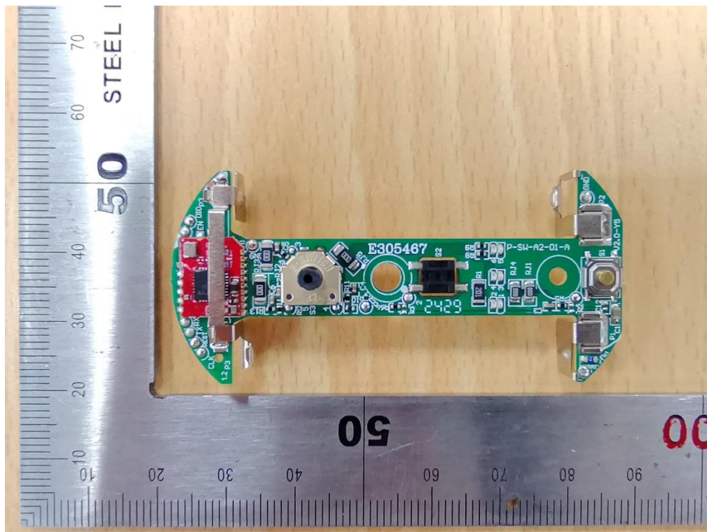
Bild / Picture 4: PCB view
