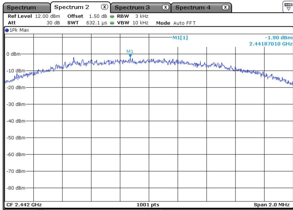
BLE_2Mbps
