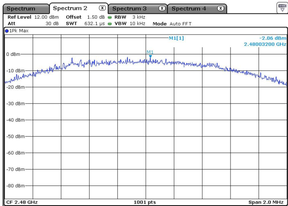
BLE_2Mbps
