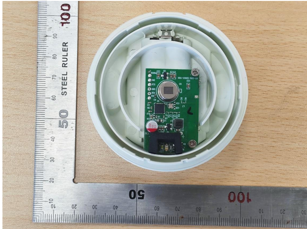
Bild / Picture 3: Internal view
