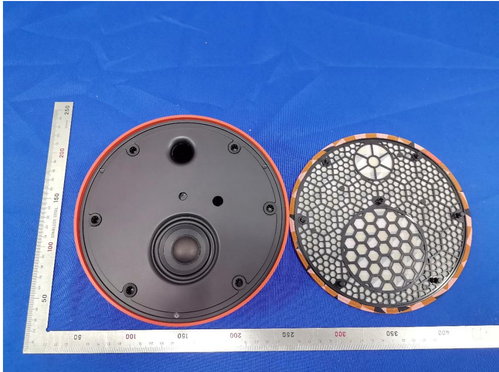
Bild / Picture 2: Internal view
