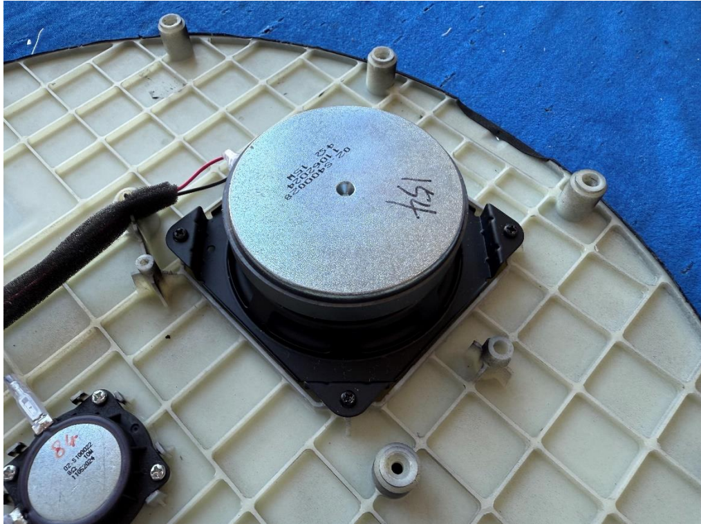
Bild / Picture 10: Tweeter view
