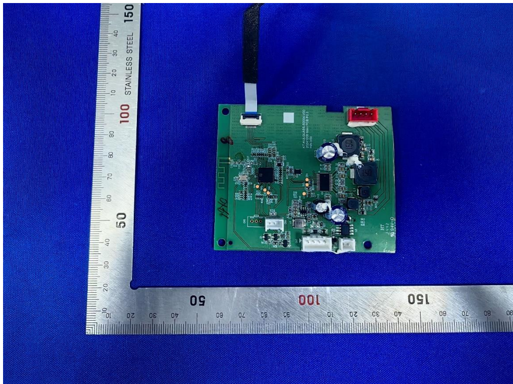
Bild / Picture 12: Mainboard view
