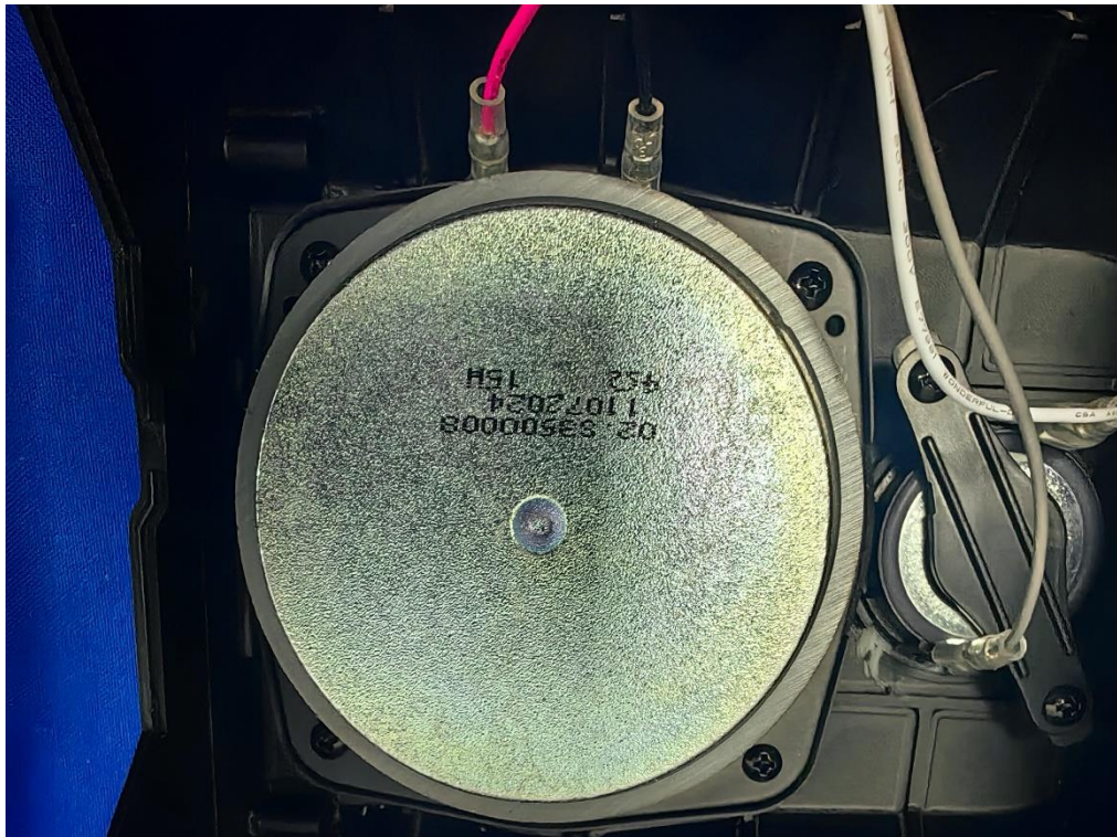
Bild / Picture 10: Woofer view
