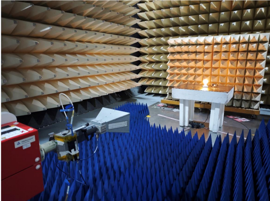
(1-18 GHz)
