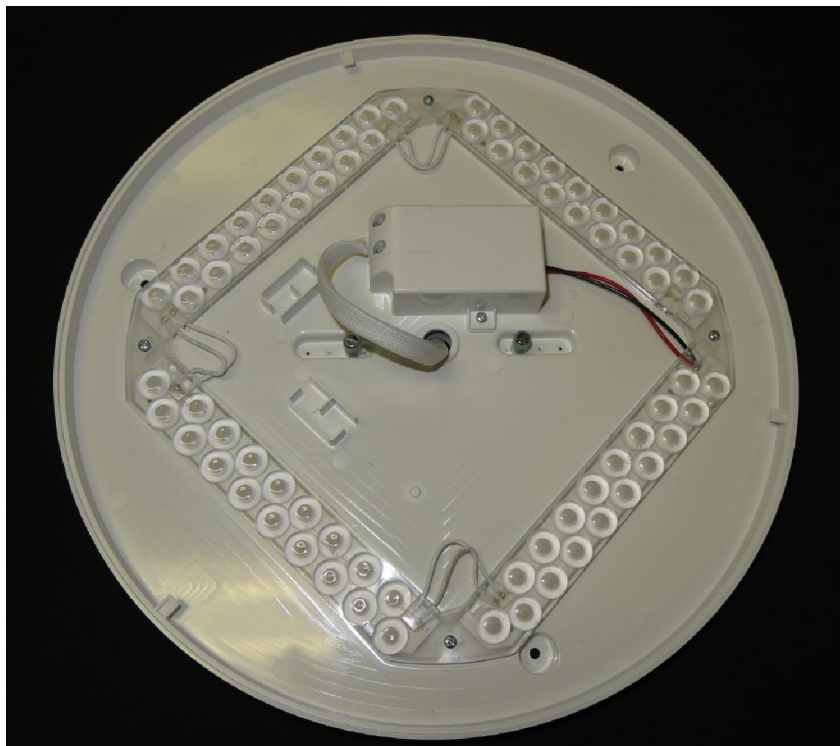
EUT
