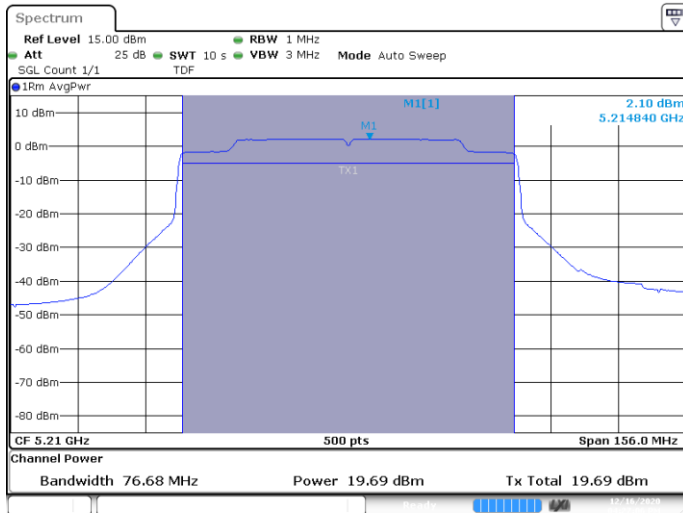
SISO A-802.11ax-80MHz-Ch42-5210MHz-HE0
