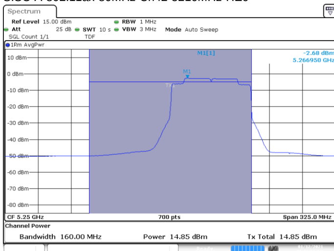
MIMO A-802.11ax-160MHz-Ch50-5250MHz-HE0-996/S67
