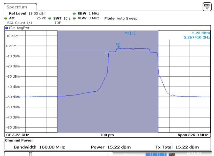
MIMO B-802.11ax-160MHz-Ch50-5250MHz-HE0-996/S67
