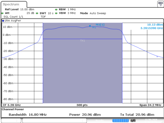
SISO B-802.11a-20MHz-Ch56-5280MHz-6
