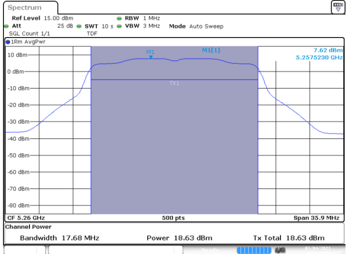
MIMO B-802.11n-20MHz-Ch52-5260MHz-HT8
