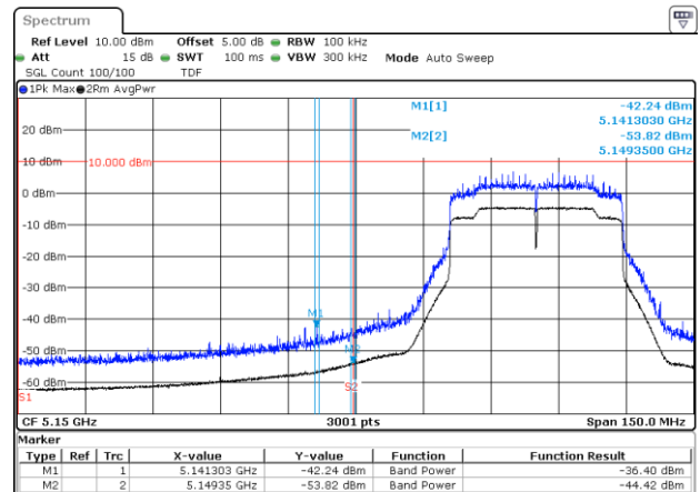
BE-R-LOW, MIMO-B, 802.11ax40-HE0, Ch38
