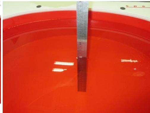
HSL(3500MHz)
