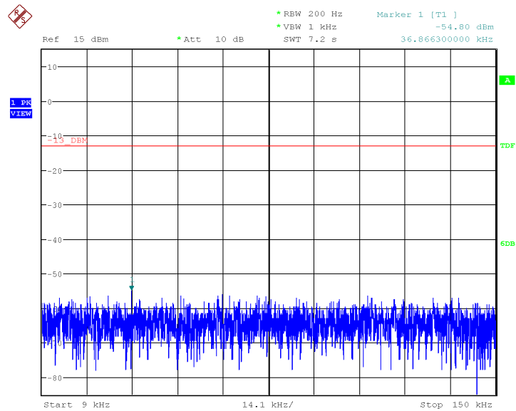
spur_8k10f1e_959.90625_9k150k.png
