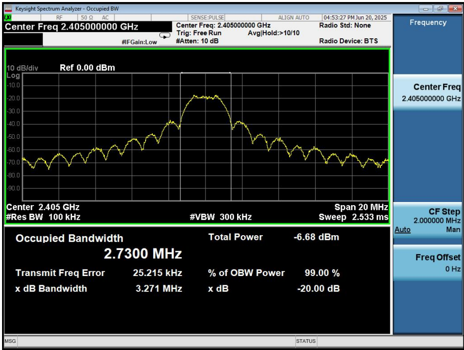
2405MHz
