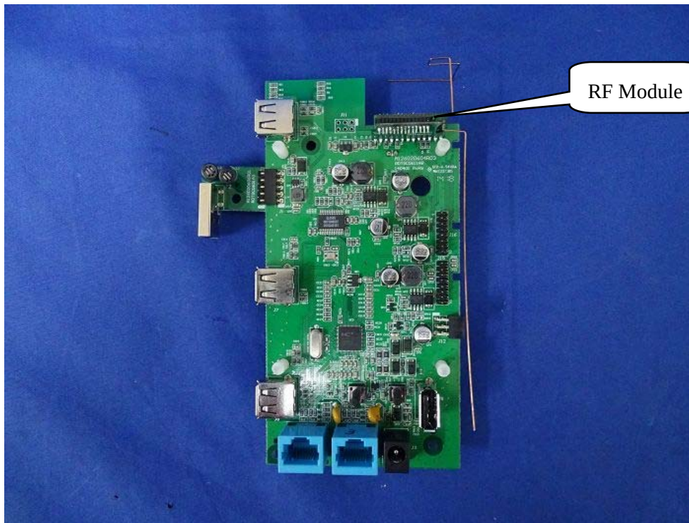
(24) EUT Photo
