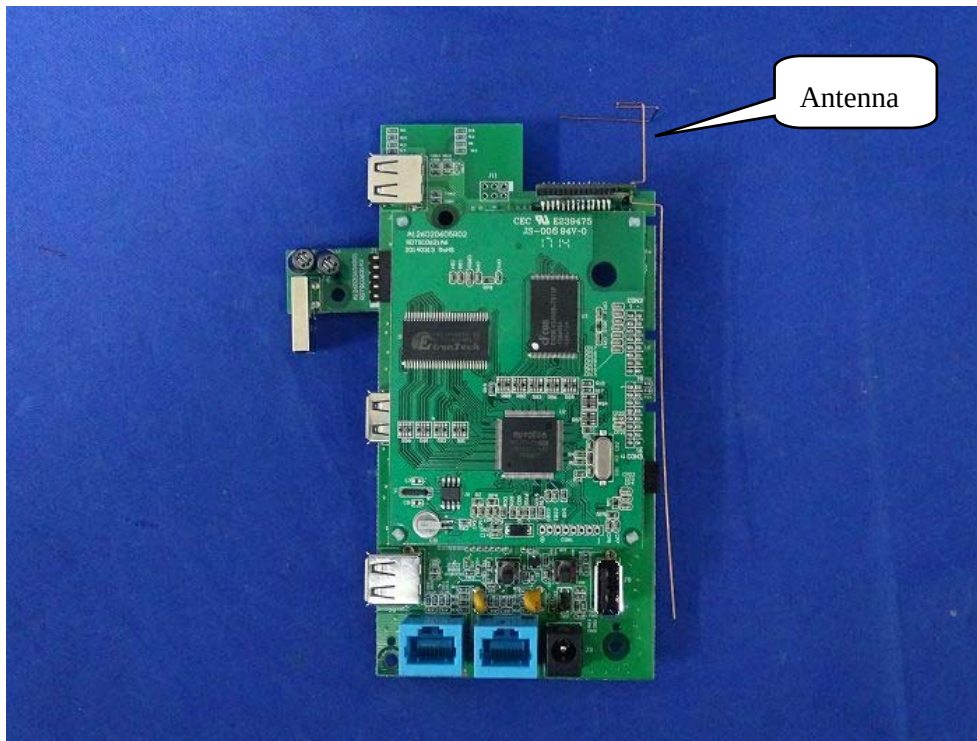
(20) EUT Photo
